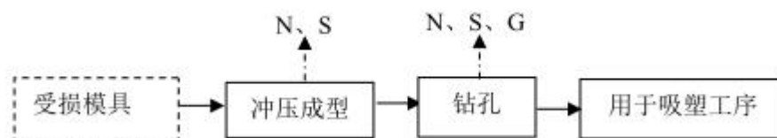
图 3-4 项目模具维修生产工艺及产污环节图
