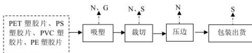
图 3-2 项目电子包装材料生产工艺及产污环节图
