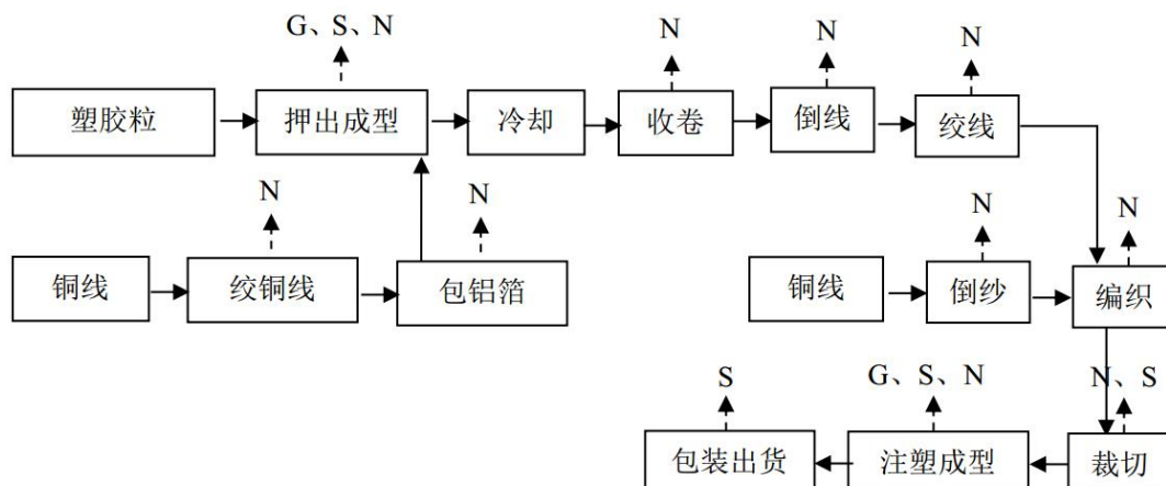
图 3-3 电线生产工艺及产污环节流程图
